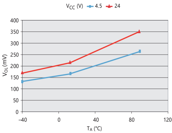
低电平(输出导通) VS 环境温度
